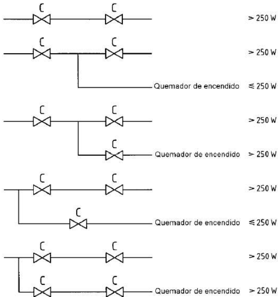
Figura G.3 - Consumos caloríficos hasta 70 kW
