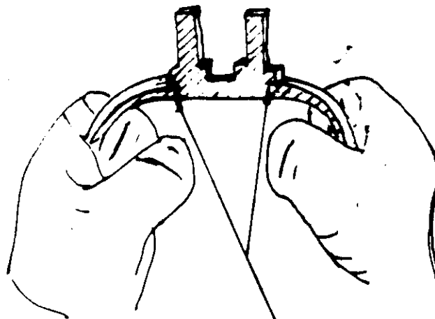
FIGURA 26.B. - DOBLADO DE LA PROBETA
