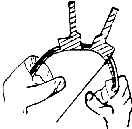
FIGURA 26.A. - AREA CIRCULAR DE FUSION SOBRE EL TUBO (IMPRONTA) INCOMPLETA
