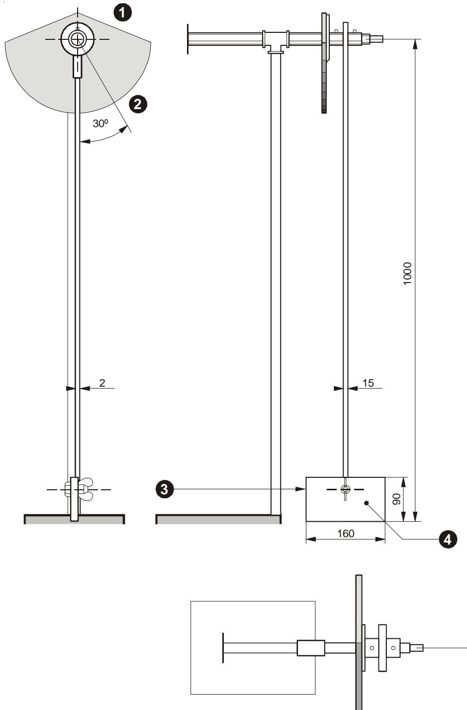
FIG. 7 - PÉNDULO PARA LOS ENSAYOS DE RESISTENCIA A LAS CORRIENTES DE AIRE DE LOS QUEMADORES DE LA ENCIMERA (APARTADO 5.3.2.2)
