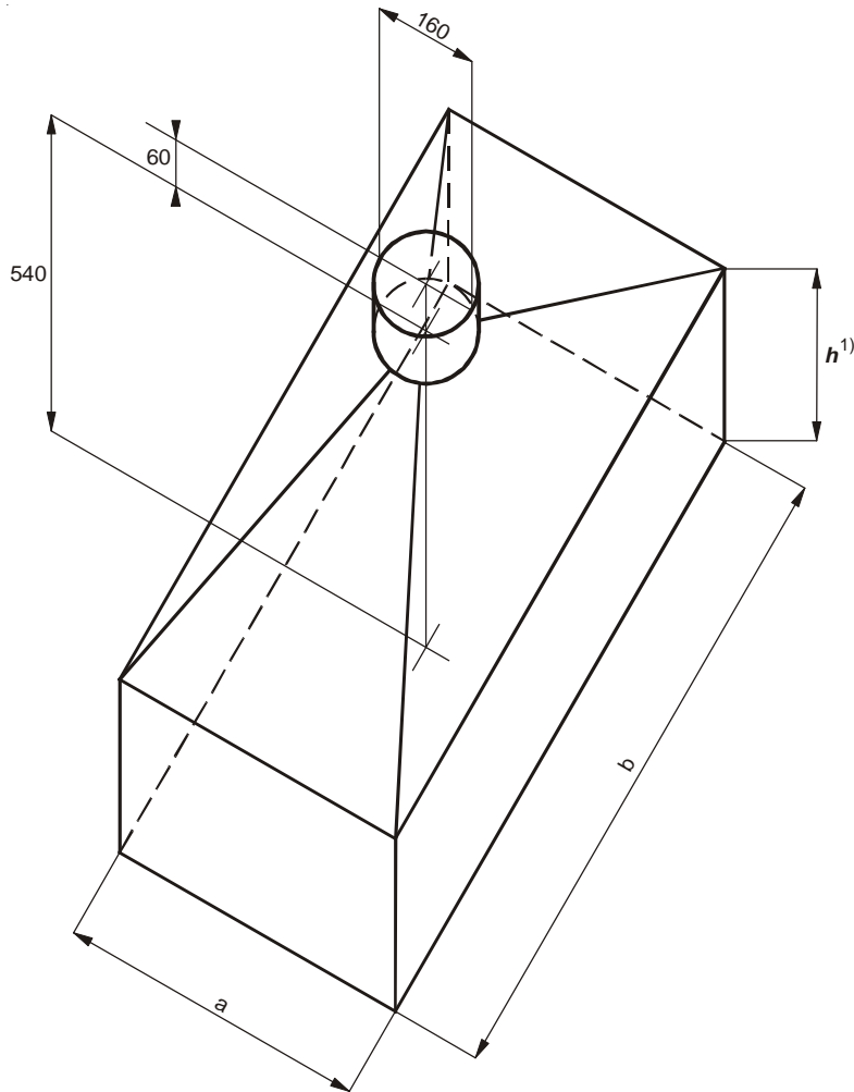
FIG. 9 - VERIFICACIÓN DE LA COMBUSTIÓN DEL CONJUNTO DE LOS QUEMADORES. DISPOSITIVO DE TOMA DE MUESTRAS (APARTADO 5.3.2.4.2)
