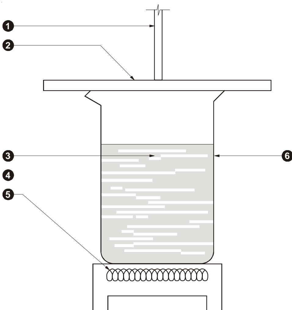
FIG. B.2 - ESQUEMA DE LOS MEDIOS DE ENSAYO PARA LA VALIDACIÓN DE LA SONDA DE TEMPERATURA DE CONTACTO
