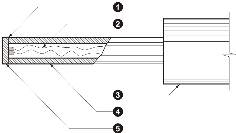
FIG. B.1 - SONDA DE TEMPERATURA DE LA SUPERFICIE
