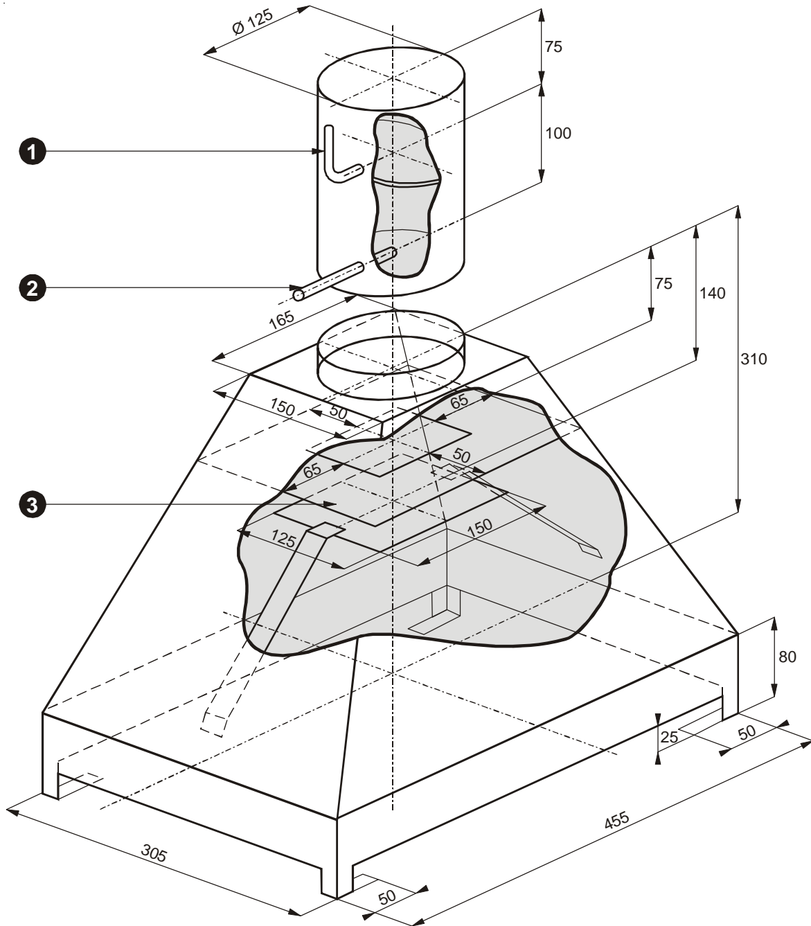
FIG. 10 - CAMPANA DE TOMA DE MUESTRAS PARA LOS GRATINADORES ELEVADOS (APARRADOS 5.3.3.2.1 Y 5.3.3.2.6)
