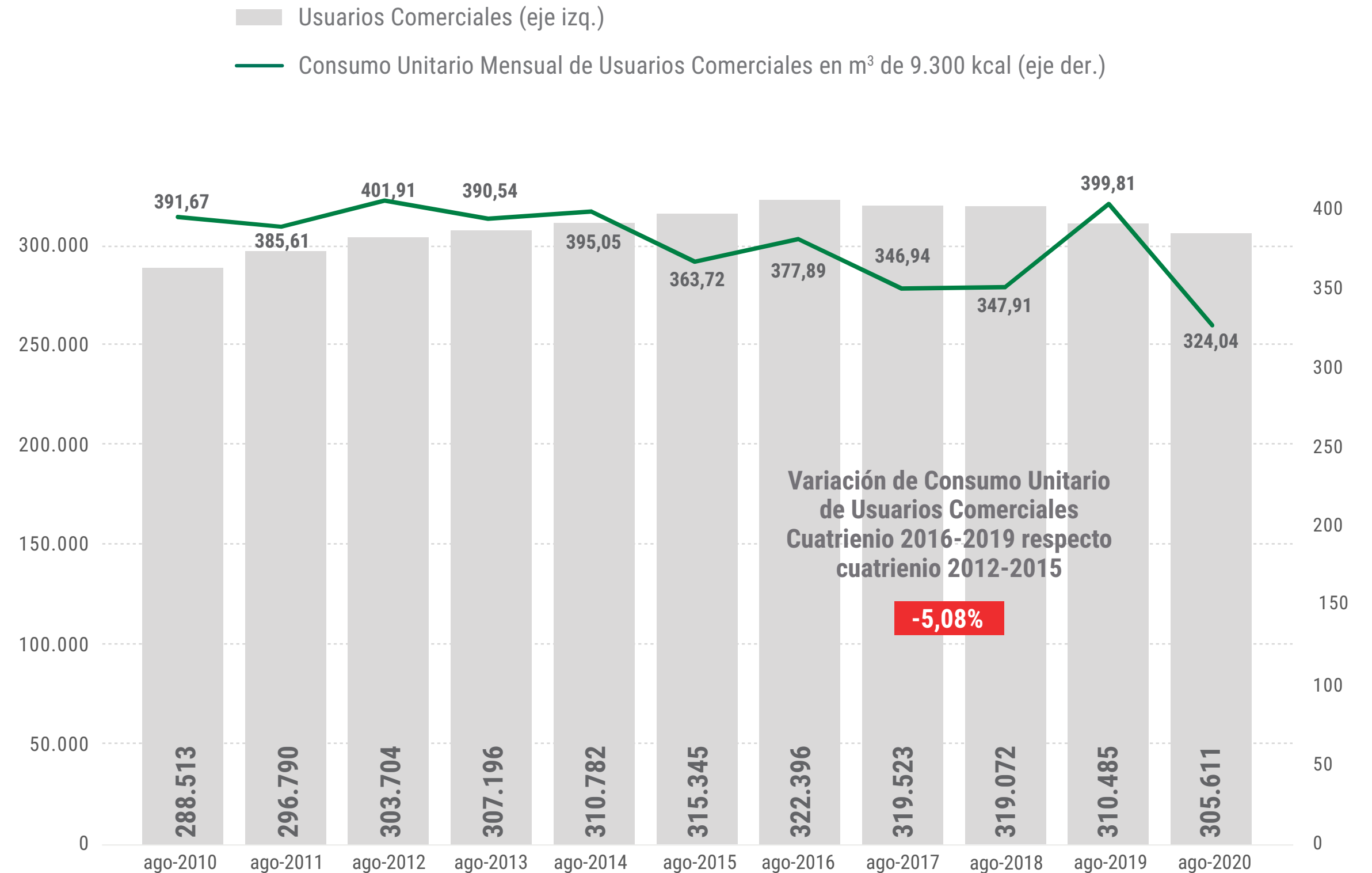
Usuarios comerciales (agosto) y consumo unitario mensual de gas natural en Argentina (promedio enero-agosto 2010-2020)
