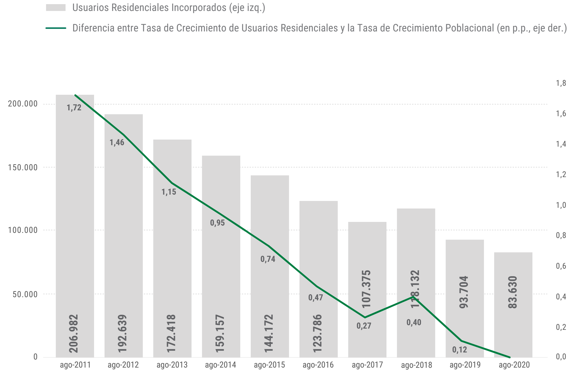
Cantidad de usuarios residenciales incorporados a la red y diferencia entre su tasa de crecimiento y la tasa de crecimiento poblacional. Mes de agosto 2011-2020
