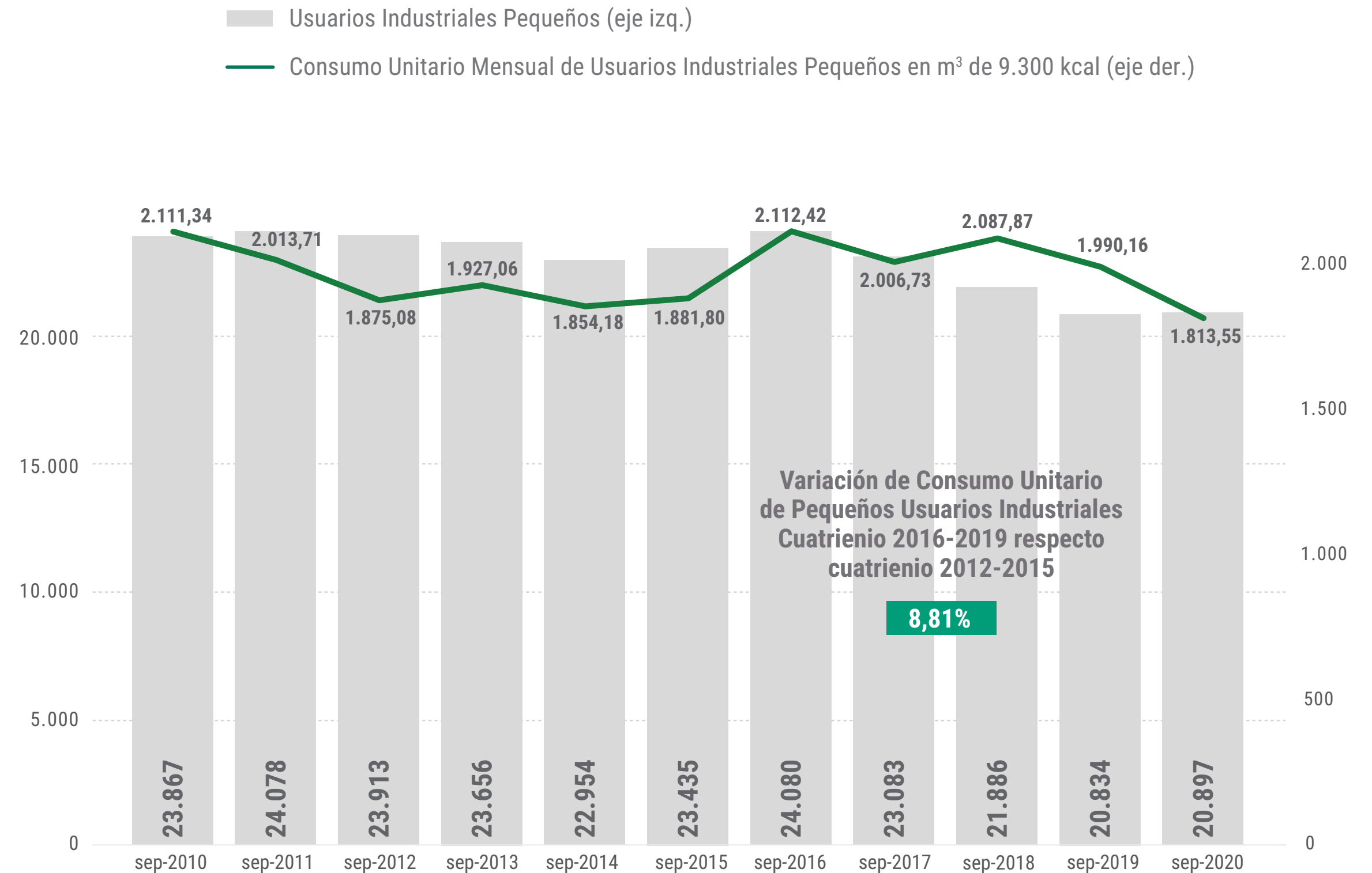
Usuarios industriales pequeños (septiembre) y consumo unitario mensual de gas natural en Argentina (promedio enero-septiembre 2010-2020)
