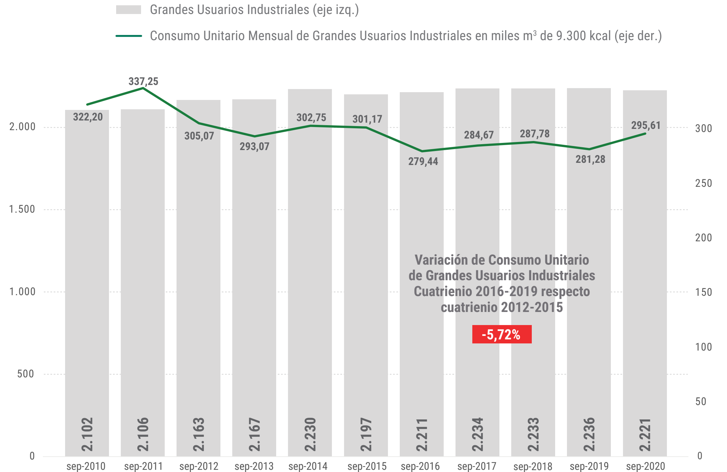
Grandes usuarios industriales (septiembre) y consumo unitario promedio de gas natural en Argentina (enero-septiembre 2010-2020)
