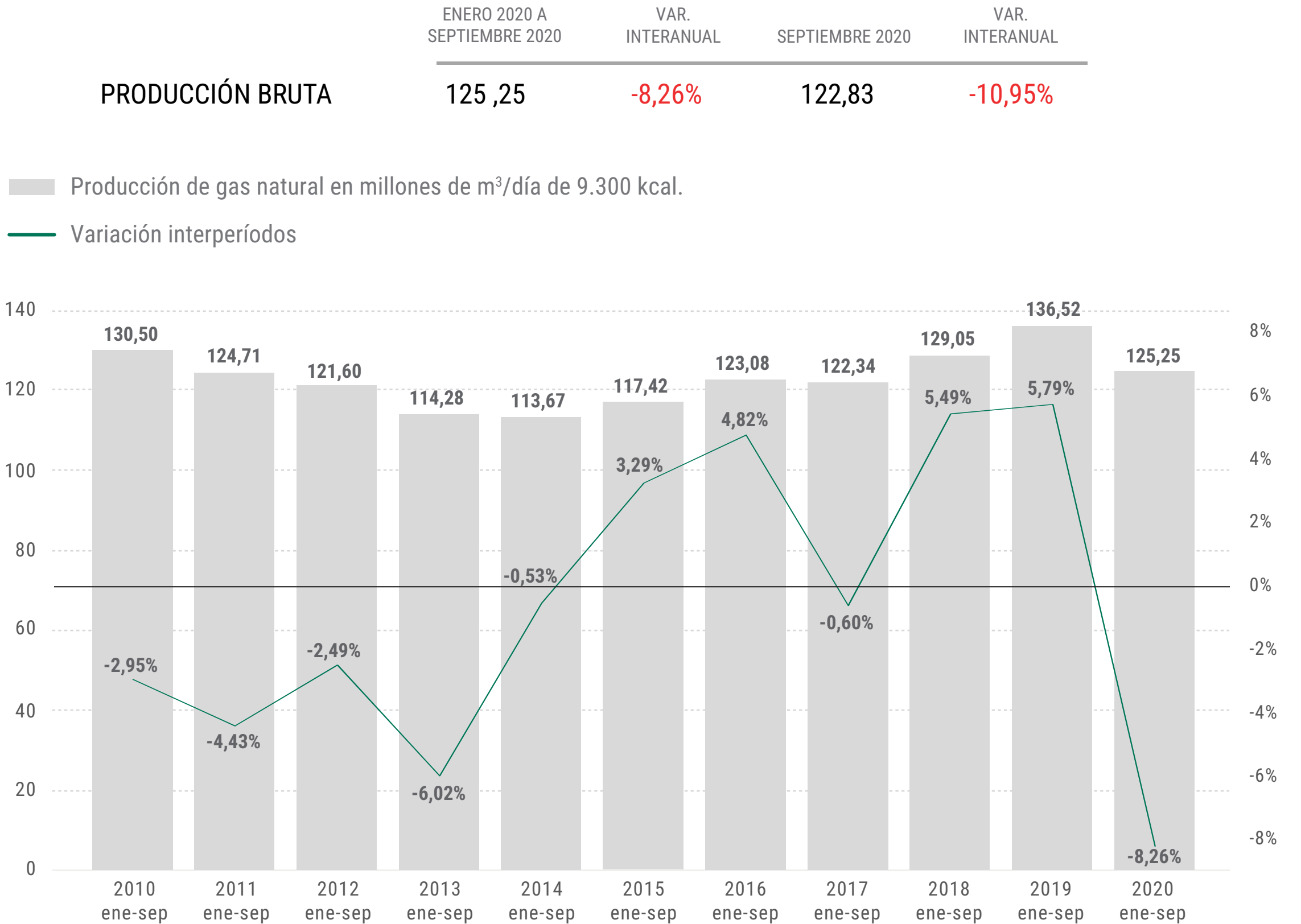
Producción bruta de gas natural en Argentina. En millones de m 3 /día de 9.300 kcal. Enero a Septiembre 2010-2020
